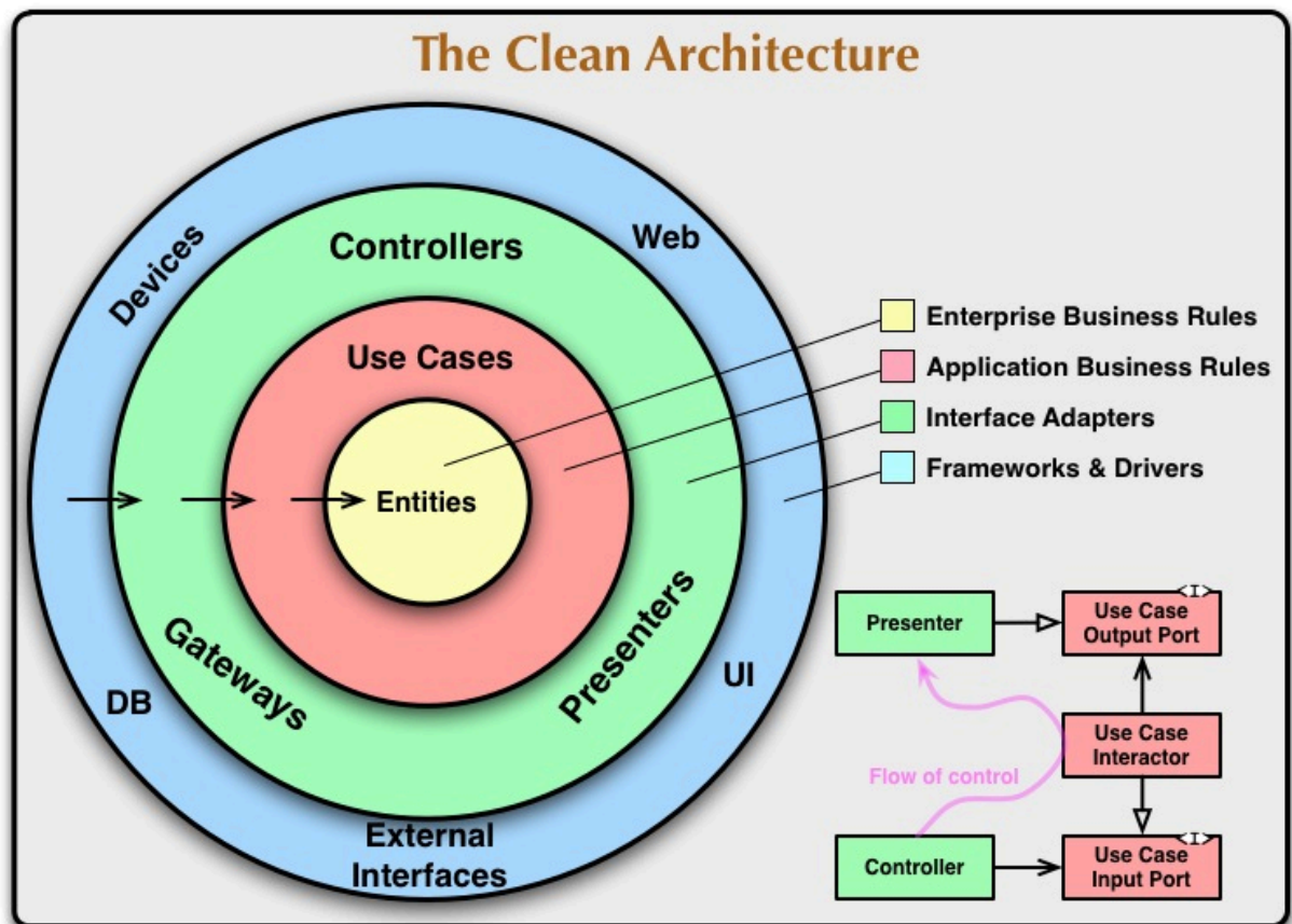
Рис. 11. Чистая архитектура
